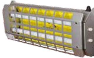
ST 519 Sinek Tutucu, Paslanmaz Çelik Fly Holder, Stainless Steel Etki Alanı / Area of Influence : 300 m 2 Ağırlık / Weight : 7,6 kg Ölçüler / Size : 129 x 35 x 95 cm
