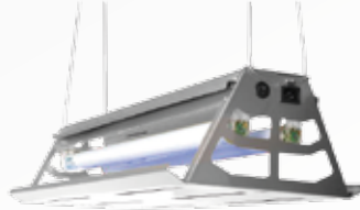
ST 516 Sinek Tutucu, Paslanmaz Çelik Fly Holder, Stainless Steel Etki Alanı / Area of Influence : 120-240 m 2 Ağırlık / Weight : 3,7 kg - Ölçüler / Size : 65 x 19 x 30 cm
