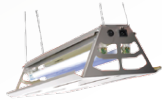
ST 517 Sinek Tutucu, Paslanmaz Çelik Fly Holder, Stainless Steel Etki Alanı / Area of Influence : 300 m 2 Ağırlık / Weight : 7,1 kg - Ölçüler / Size : 129 x 19 x 30 cm
