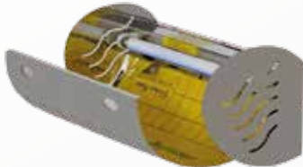
ST 524 Sinek Tutucu, Paslanmaz Çelik Fly Holder, Stainless Steel Etki Alanı / Area of Influence : 20 - 30 m 2 Ağırlık / Weight : 1,8 kg Ölçüler / Size : 33,5 x 14,5 x 16 cm
